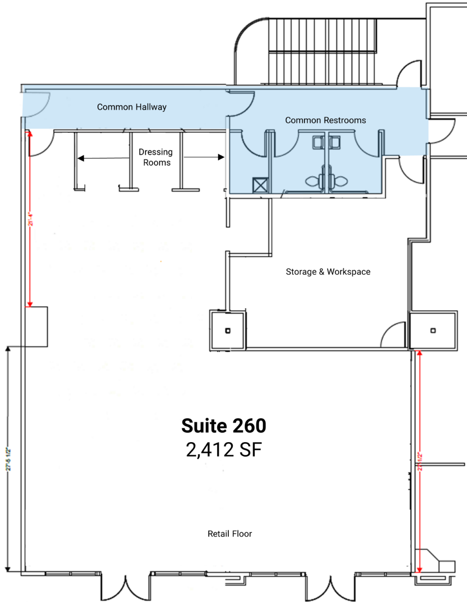
FLOOR PLAN Scale: 1/8" = 1'
